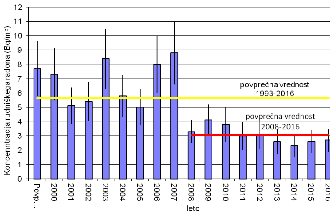
Slika 5: Prispevek rudniškega Rn-222 k celotni koncentraciji Rn-222 v okolju
