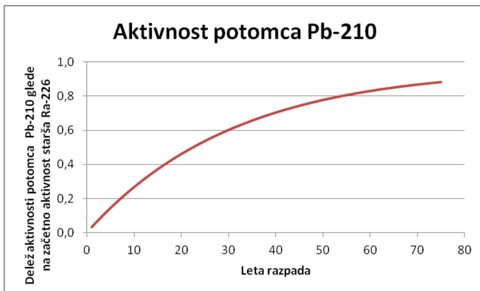
Slika 10: Povečevanje aktivnosti Pb-210 zaradi radiaktivnega razpada Ra-226.
