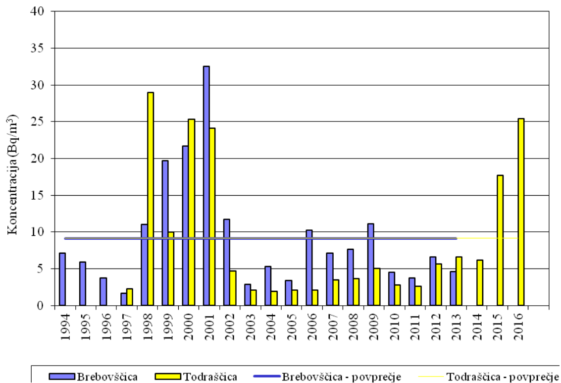
Slika 9: Povprečne letne koncentracije Pb-210 v Brebovšičici in Todraščici PO
