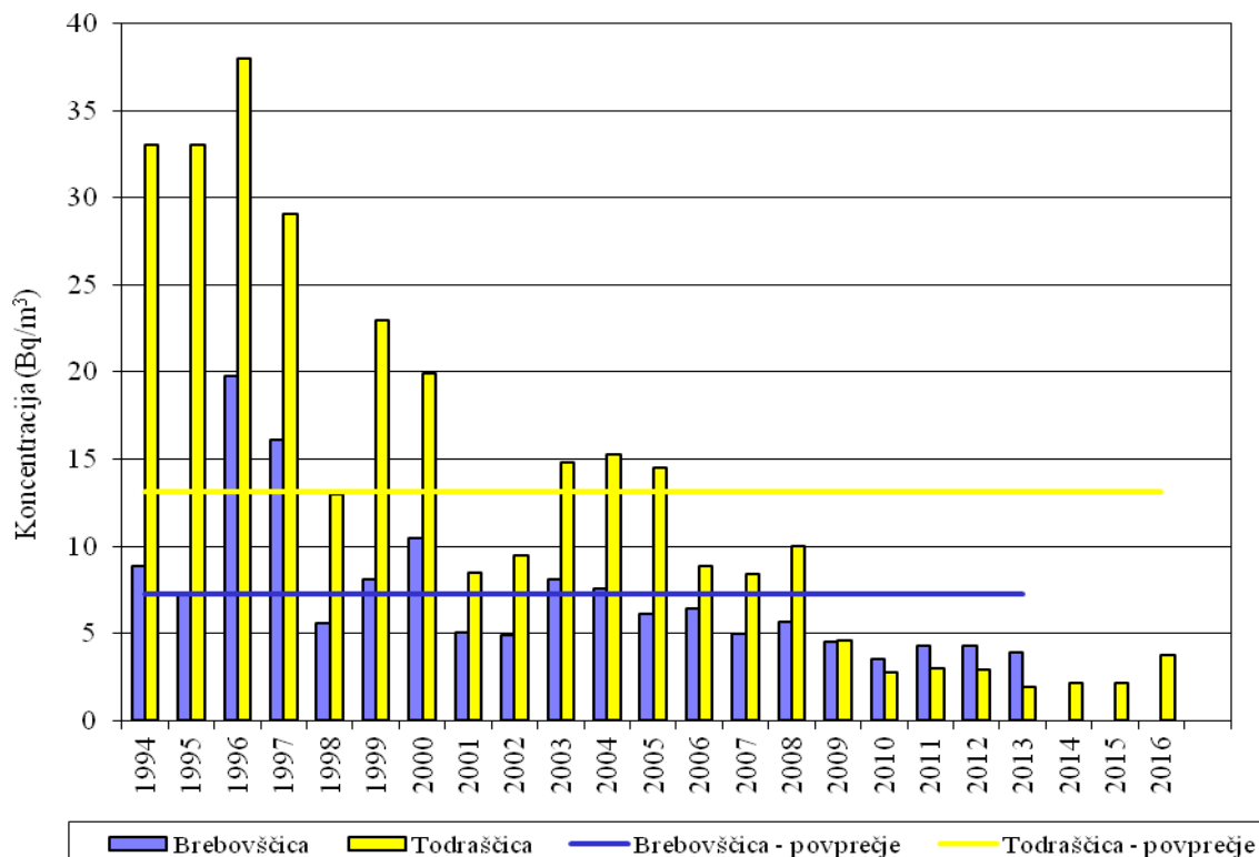
Slika 8: Povprečne letne koncentracije Ra-226 v Brebovšičici in Todraščici PO
