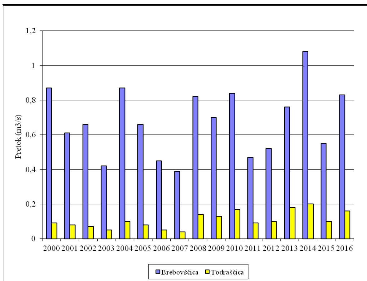
Slika 11: Povprečni pretoki v Brebovščici in Todraščici
