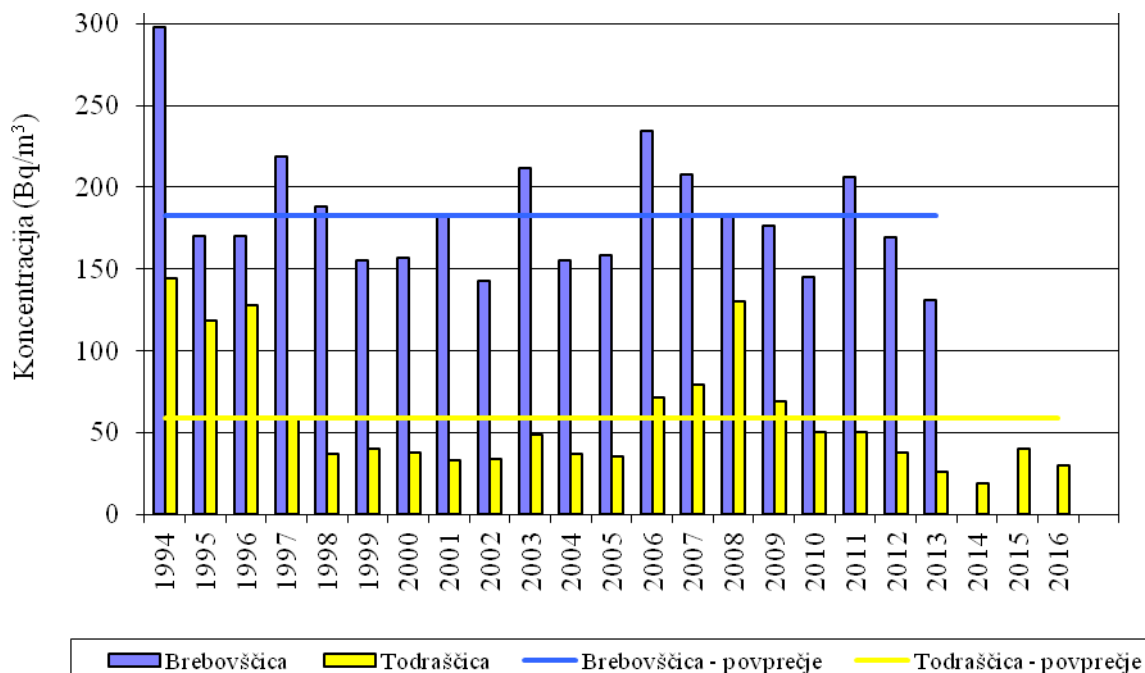
Slika 7: Povprečne letne koncentracije U-238 v Brebovščici in Todraščici PO
