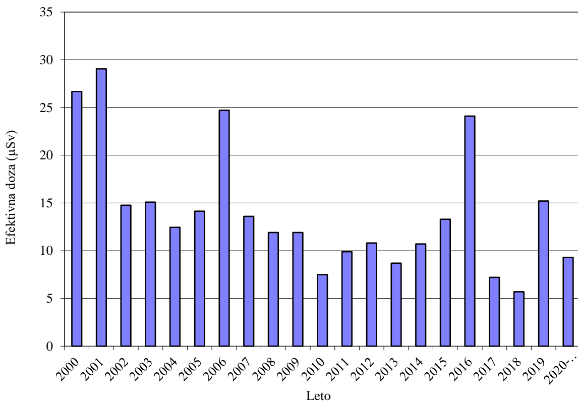
Slika 18: Letne efektivne doze zaradi pitja vode za odraslega prebivalca iz okolice RŽV. Do leta 2019 so ocenjeni prispevki zaradi pitja Brebovščice, za 2020 pa zaradi pitja Todraščice.
