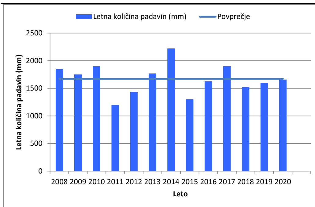
Slika 1: Letne količine padavin (mm) na vremenski postaji Boršt.
