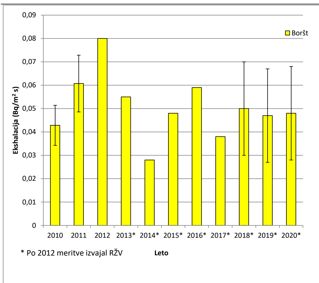
Slika 4: Ekshalacija radona iz odlagališča Boršt po izvedenih zapiralnih delih. Prikazano je povprečje letnih in zimskih meritev.
