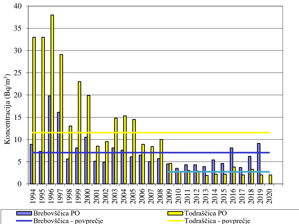
Slika 5: Povprečne letne koncentracije U-238 v Brebovščici PO in Todraščici PO. Za vrednosti v Brebovščici PO od 2014 dalje navajamo izmerjene vrednosti v enkratnem vzorcu, ki naj bi bil odvzet v času povprečnega pretoka.
