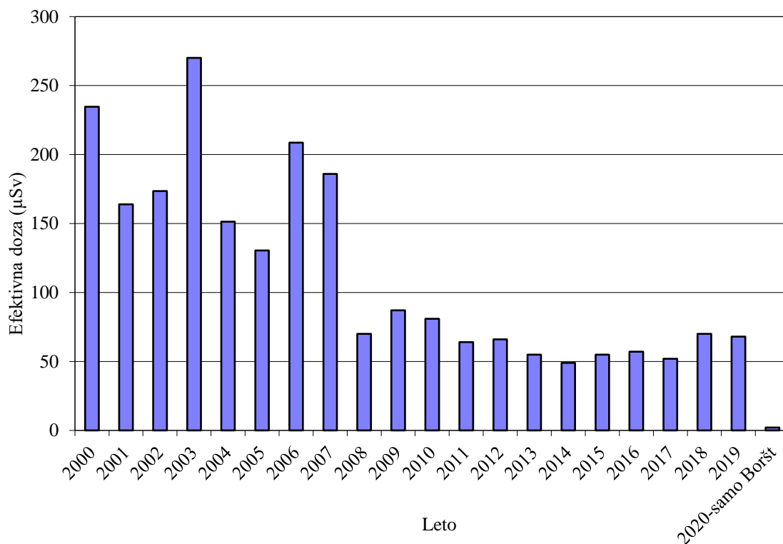
Slika 17: Efektivne letne doze zaradi vdihavanja radonovih kratkoživih potomcev za odraslega prebivalca v okolici RŽV
