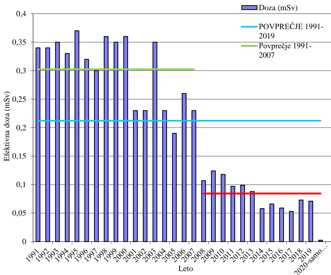
Slika 19: Skupne letne efektivne doze prebivalcev po letih zaradi vpliva RŽV. Za leto 2020 je izračunana le doza zaradi vpliva odlagališča Boršt
