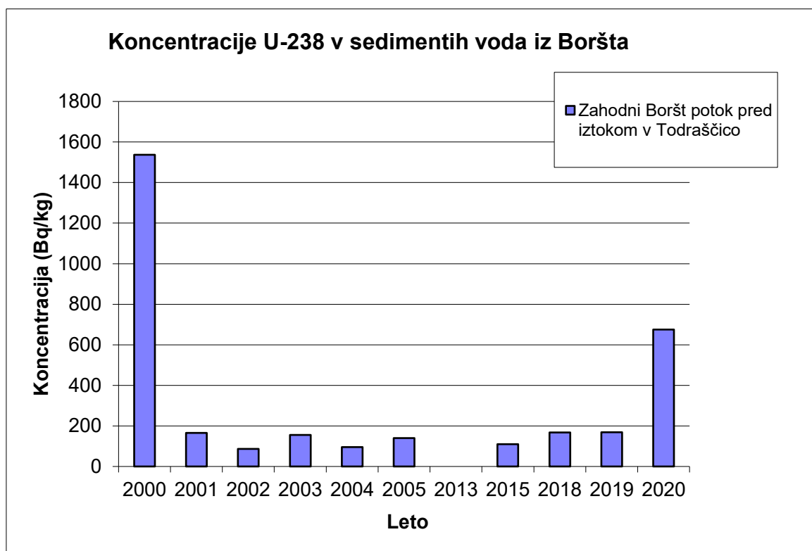
Slika 13: Koncentracije U-238 v sedimentih iz Boršta
