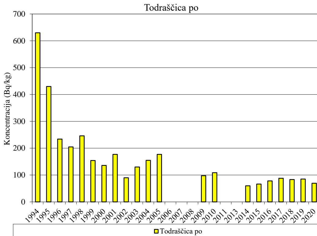
Slika 11: Koncentracija Ra-226 v sedimentih voda v Todraščici PO
