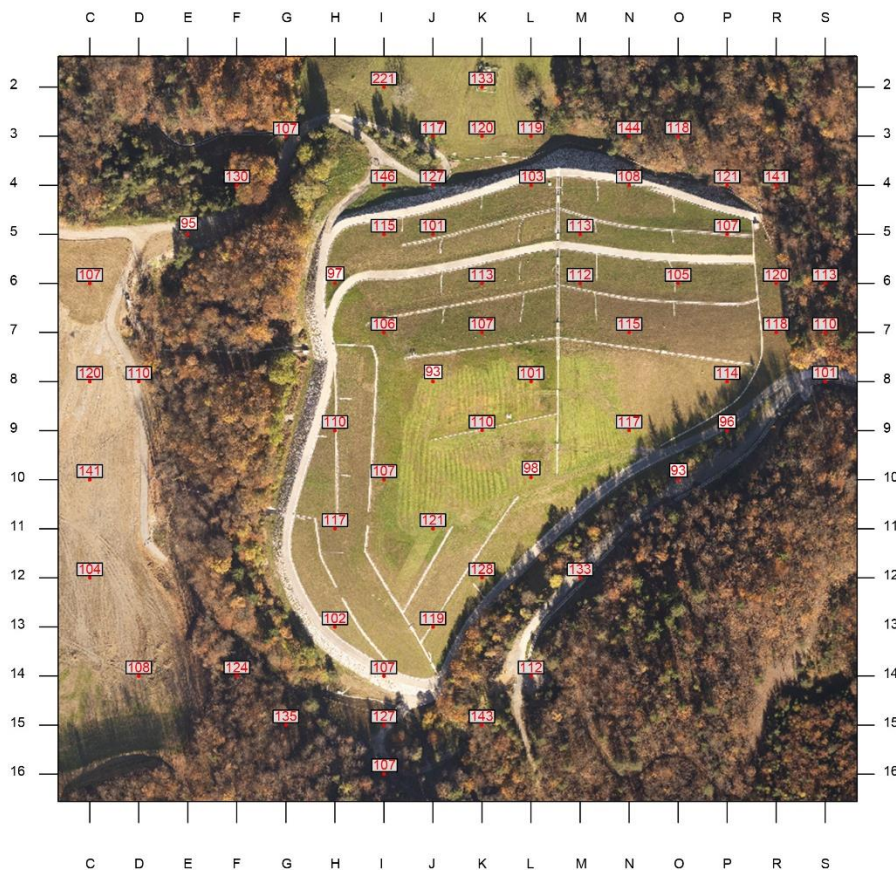
Slika 16: Meritve hitrosti doze zunanega sevanja gama na površini odlagališča Boršt. Meritve sta izvedla J. Čadež in J. Rojc iz RŽV, d.o.o.
