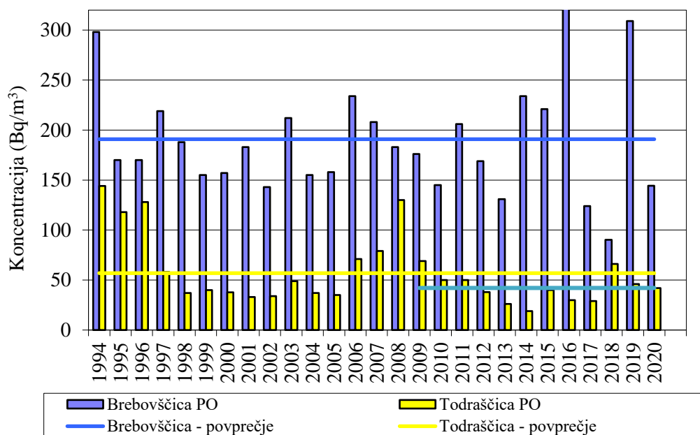
Slika 5: Povprečne letne koncentracije U-238 v Brebovščici PO in Todraščici PO. Za vrednosti v Brebovščici PO od 2014 dalje navajamo izmerjene vrednosti v enkratnem vzorcu, ki naj bi bil odvzet v času povprečnega pretoka.
