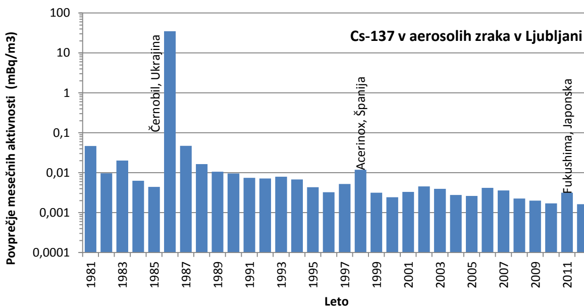
Slika 13: Povprečne mesečne specifične aktivnosti Cs-137 v zraku na lokaciji Ljubljana za obdobje od leta 1986 dalje
