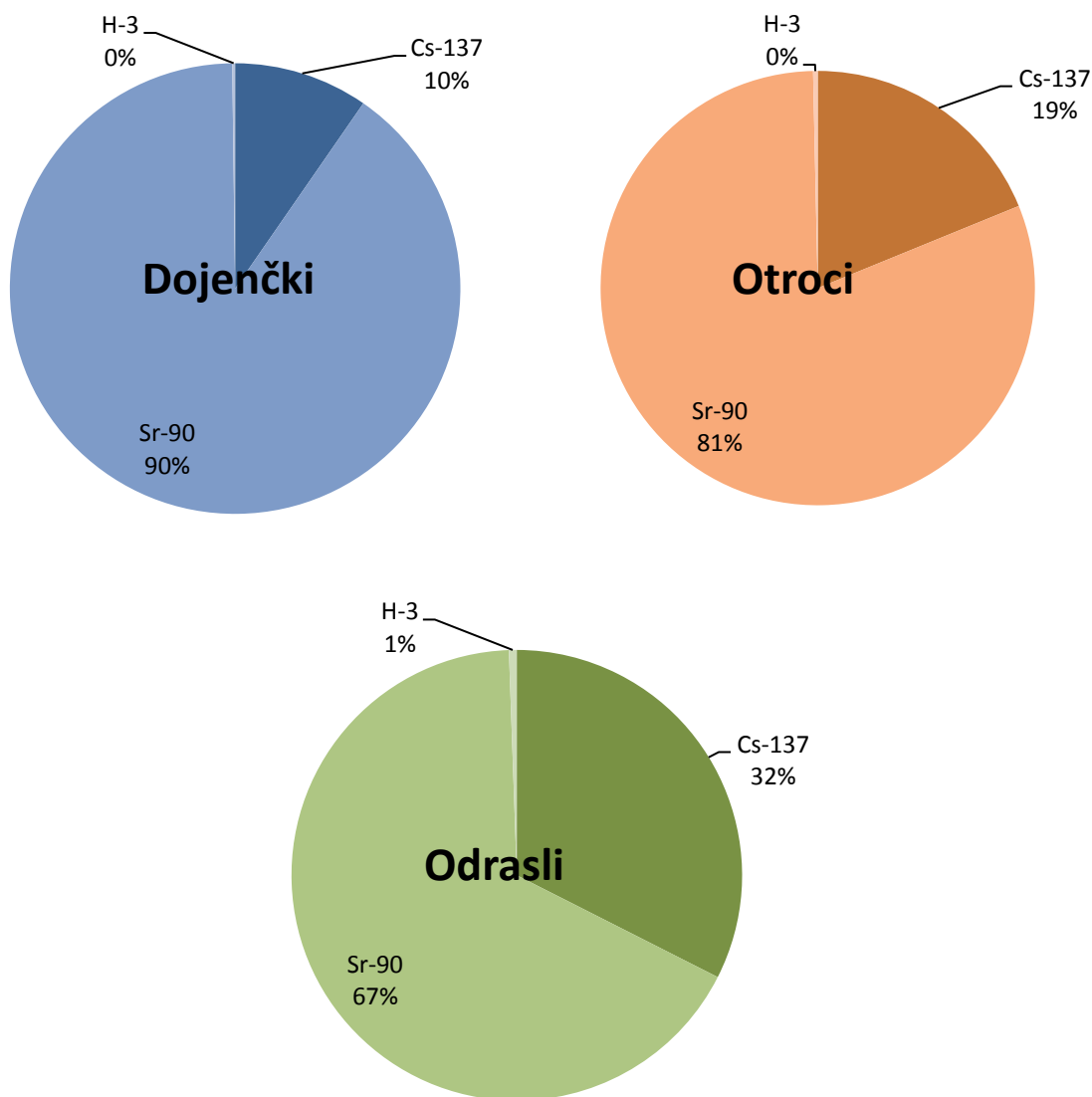
Slika 37: Relativni prispevki k dozi posameznih radionuklidov za tri starostne skupine prebivalstva (ljubljsko mleko)
