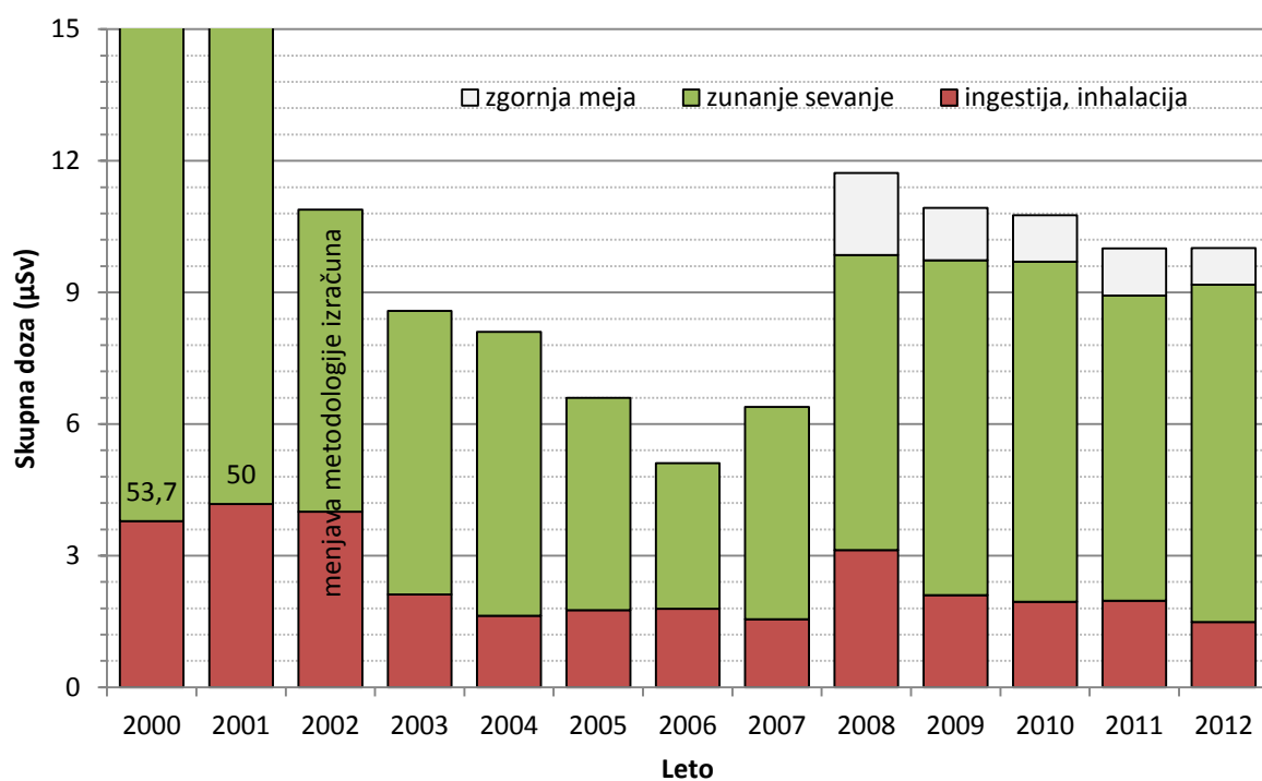
Slika 38: Predvidena efektivna doza H_E zaradi kontaminacije okolja z dolgoživimi fizijskimi radionuklidi za odrasle (slovensko povprečje) za obdobje od leta 2000 dalje
