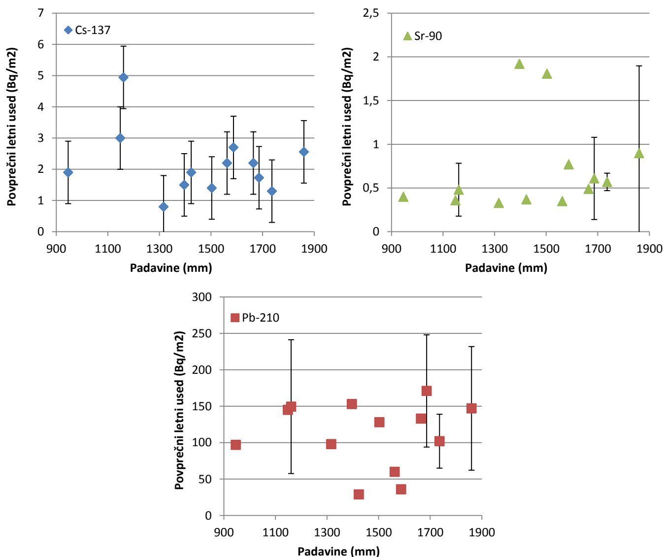
Slika 15: Korelacija količine padavin s povprečnim letnim usedom Cs-137, Sr-90 in Pb-210 na enoto površine (povprečje vseh lokacij po Sloveniji)
