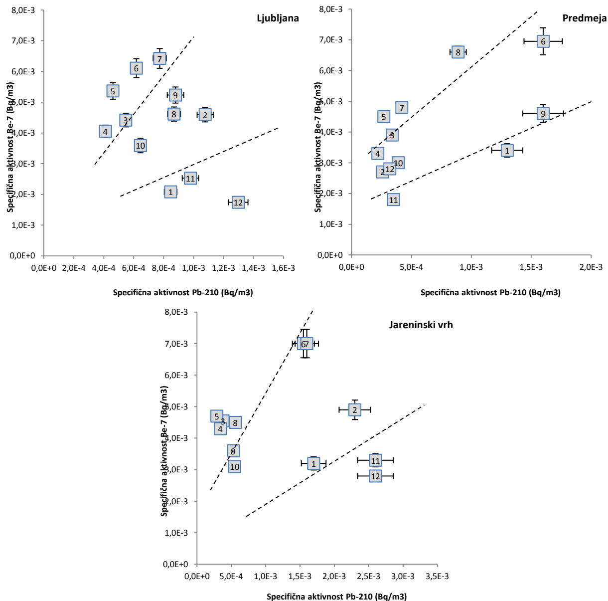
Slika 12: Zimske in poletne korelacije med izmerjenimi koncentracijami atmosferskega Pb-210 in Be-7 v zraku na različnih lokacijah v letu 2012 – številka ob meritvi pomeni mesec vzorčevanja.
