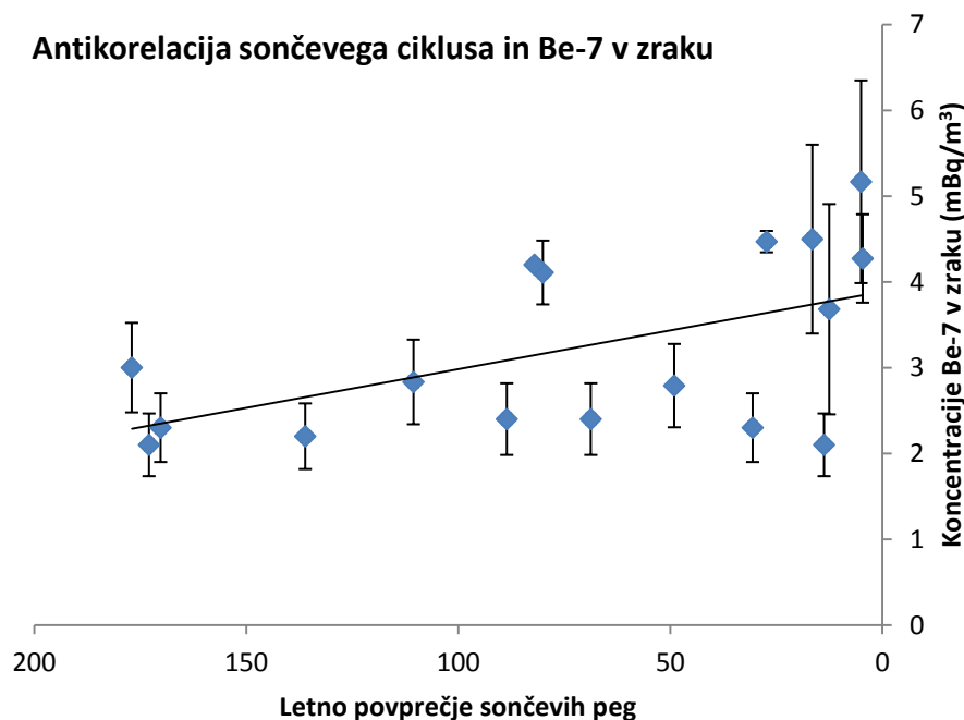
Slika 8: Antikorelacija sončevega cikla s koncentracijami Be-7 v zraku.
