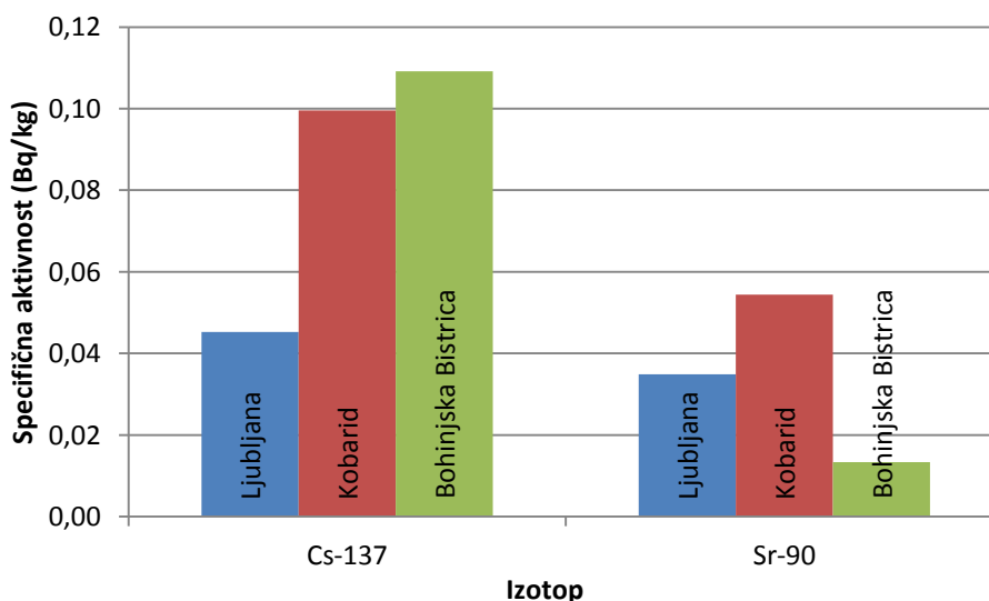
Slika 26: Primerjava povprečnih specifičnih aktivnosti Cs-137 in Sr-90 v mleku na različnih lokacijah v Sloveniji za leto 2012.
