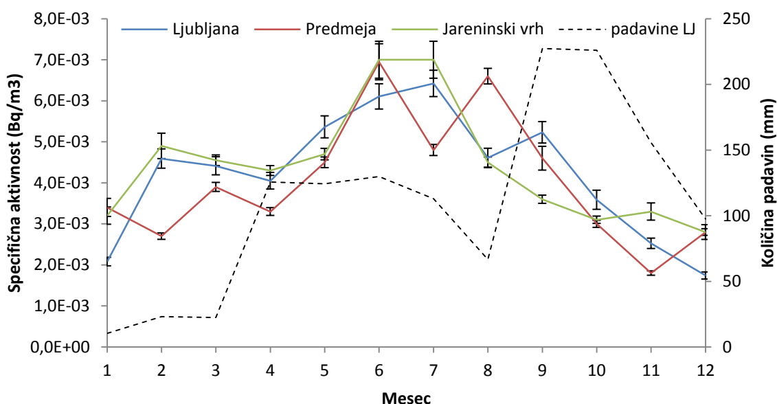
Slika 9: Sezonske variacije izmerjenih koncentracij atmosferskega Be-7 v zraku na različnih lokacijah v letu 2012
