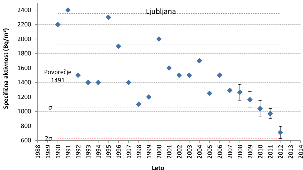
Slika 16: Specifične aktivnosti H-3 v padavinah iz Ljubljane za obdobje od leta 1990 dalje
