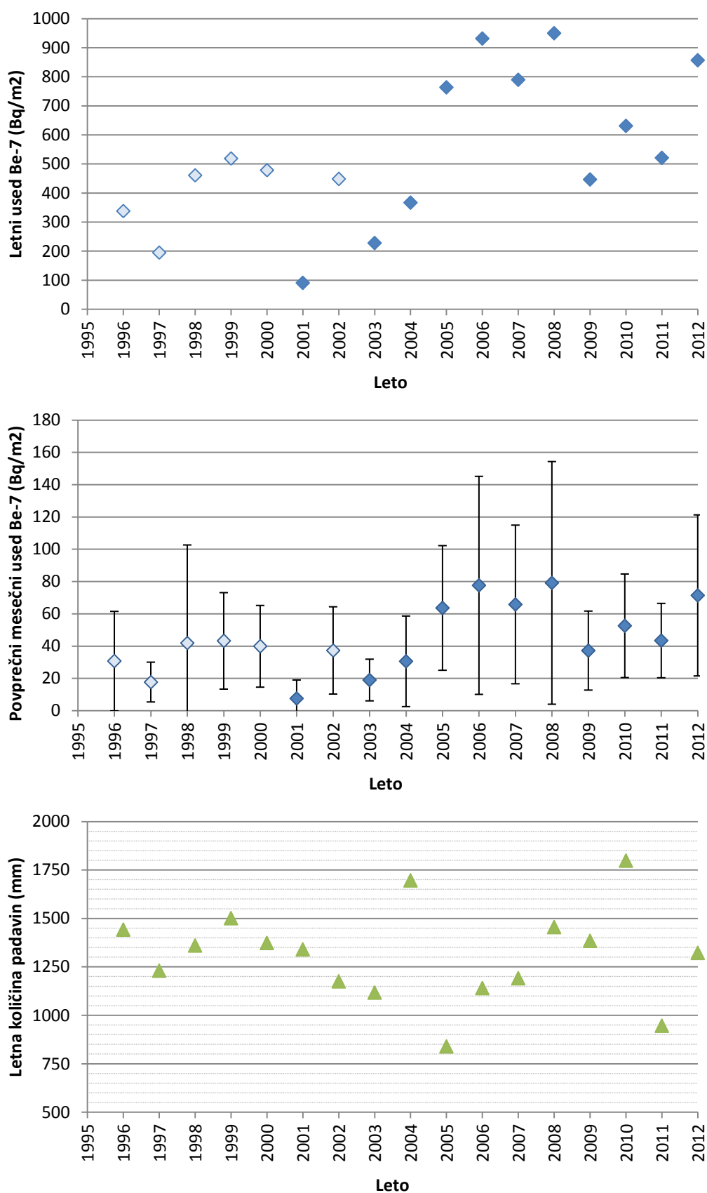
Slika 17: Specifične aktivnosti Be-7 v padavinah iz Ljubljane za obdobje od leta 1996 dalje
