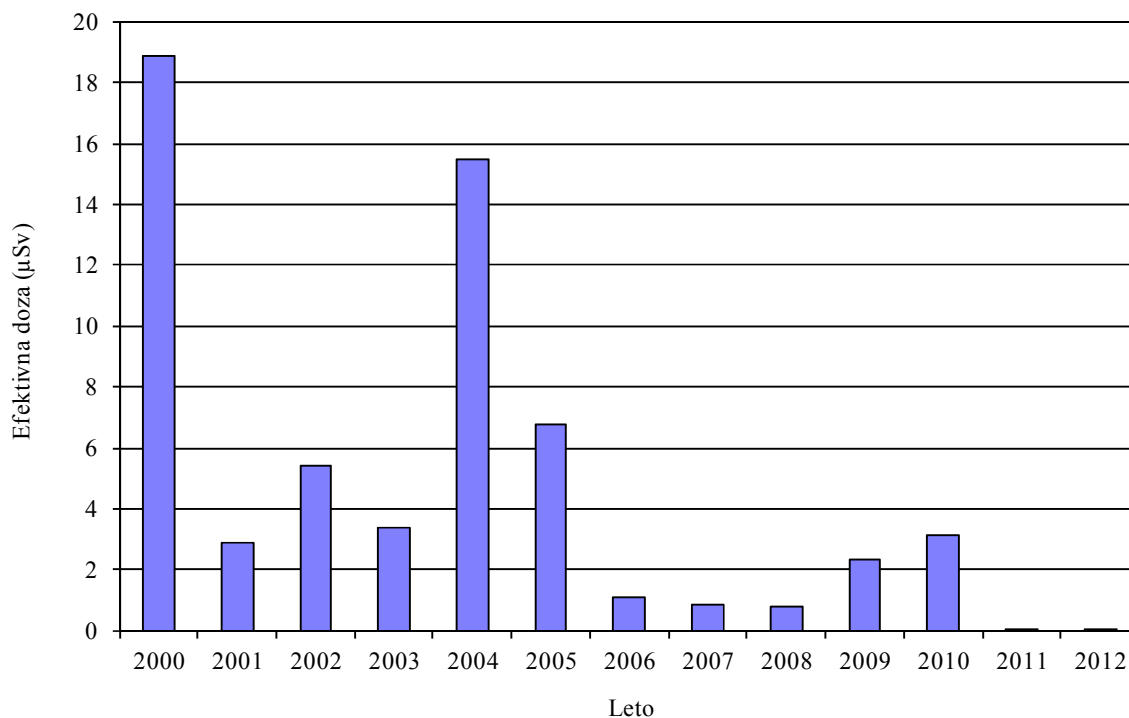
Slika 22: Letne učinkovite doze v okolici RŽV zaradi vdihavanja dolgoživih radionuklidov v zraku za odraslega prebivalca. Ocenjena letna učinkovita doza v 2012 je 0,00 µSv.
