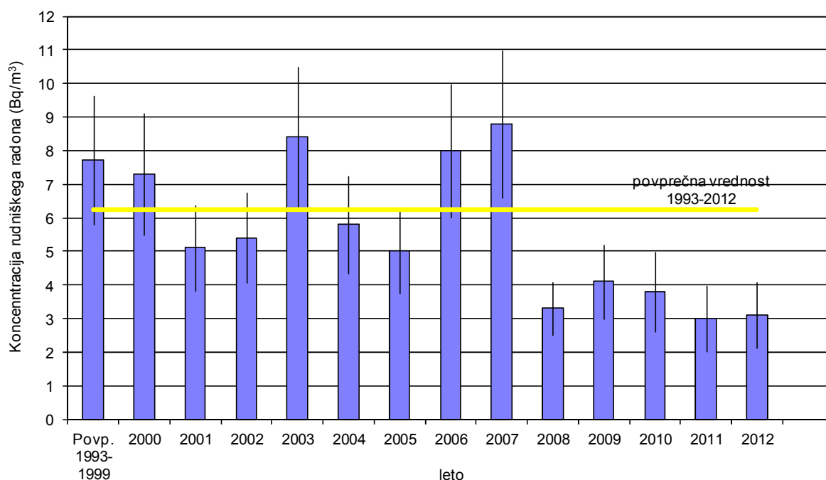
Slika 7: Prispevek rudniškega Rn-222 k celotni koncentraciji Rn-222 v okolju
