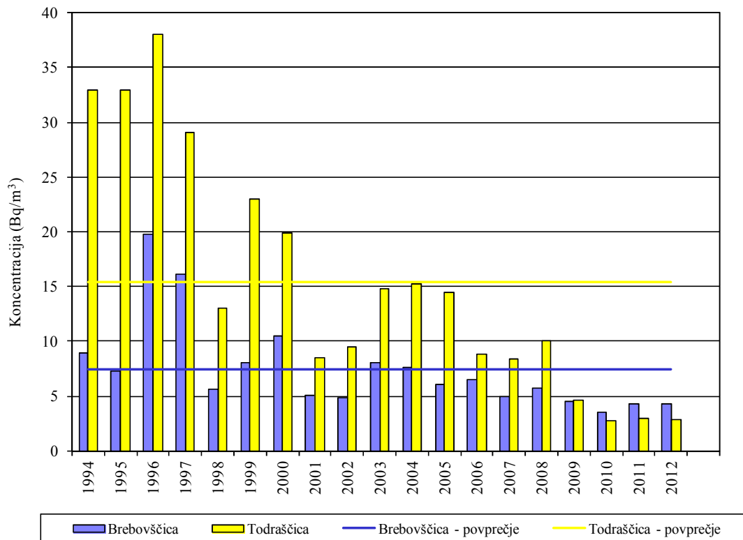
Slika 14: Povprečne koncentracije Ra-226 v Brebovščici in Todraščici
