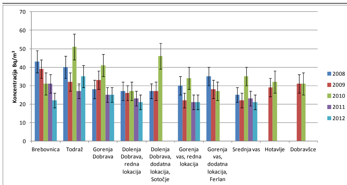
Slika 6: Koncentracije Rn-222 v dolini Brebovšče in Poljanske Sore, merjeno z detektorji sledi
