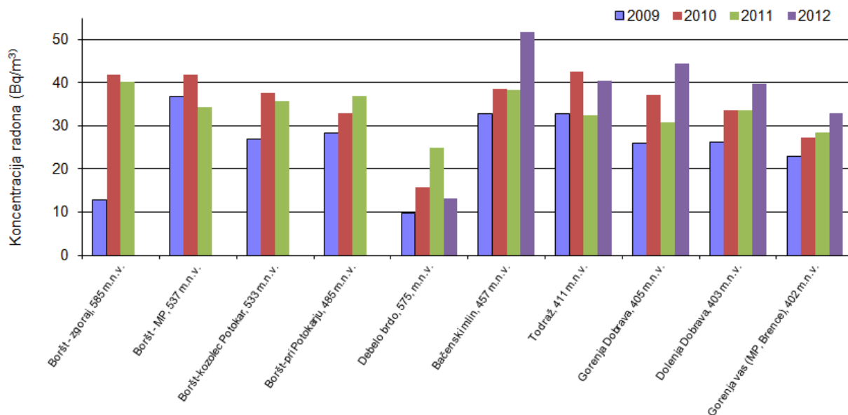
Slika 11: Višinski profil koncentracije radona po dolini Brebovščice, merjeno z ogljenimi adsorberji.
