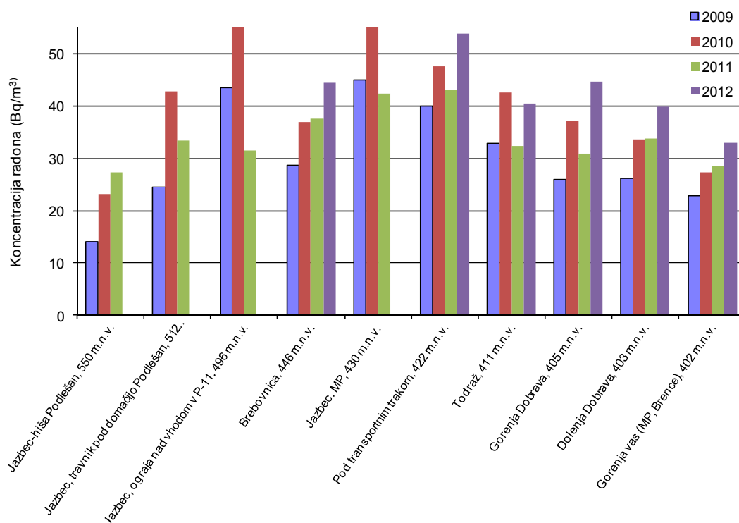
Slika 11: Višinski profil koncentracije radona po dolini Brebovščice, merjeno z ogljenimi adsorberji.
