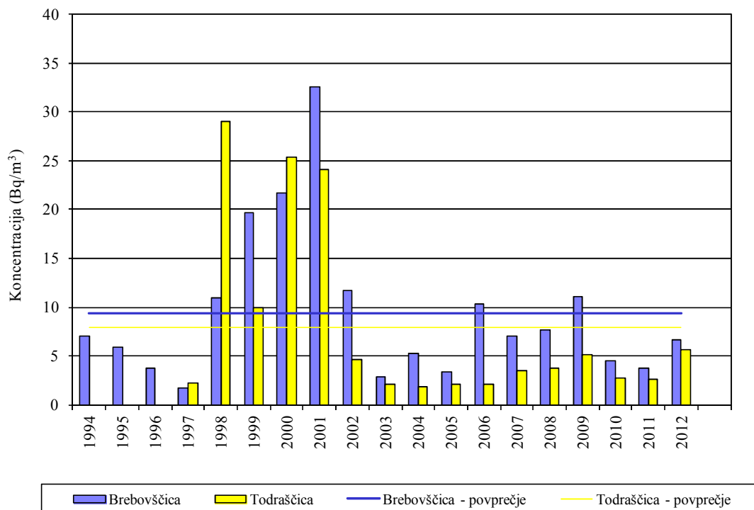
Slika 15: Povprečne koncentracije Pb-210 v Brebovščici in Todraščici
