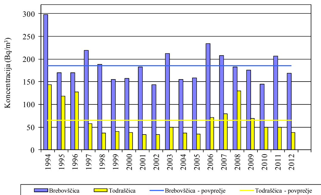
Slika 13: Povprečne koncentracije U-238 v Brebovščici in Todraščici
