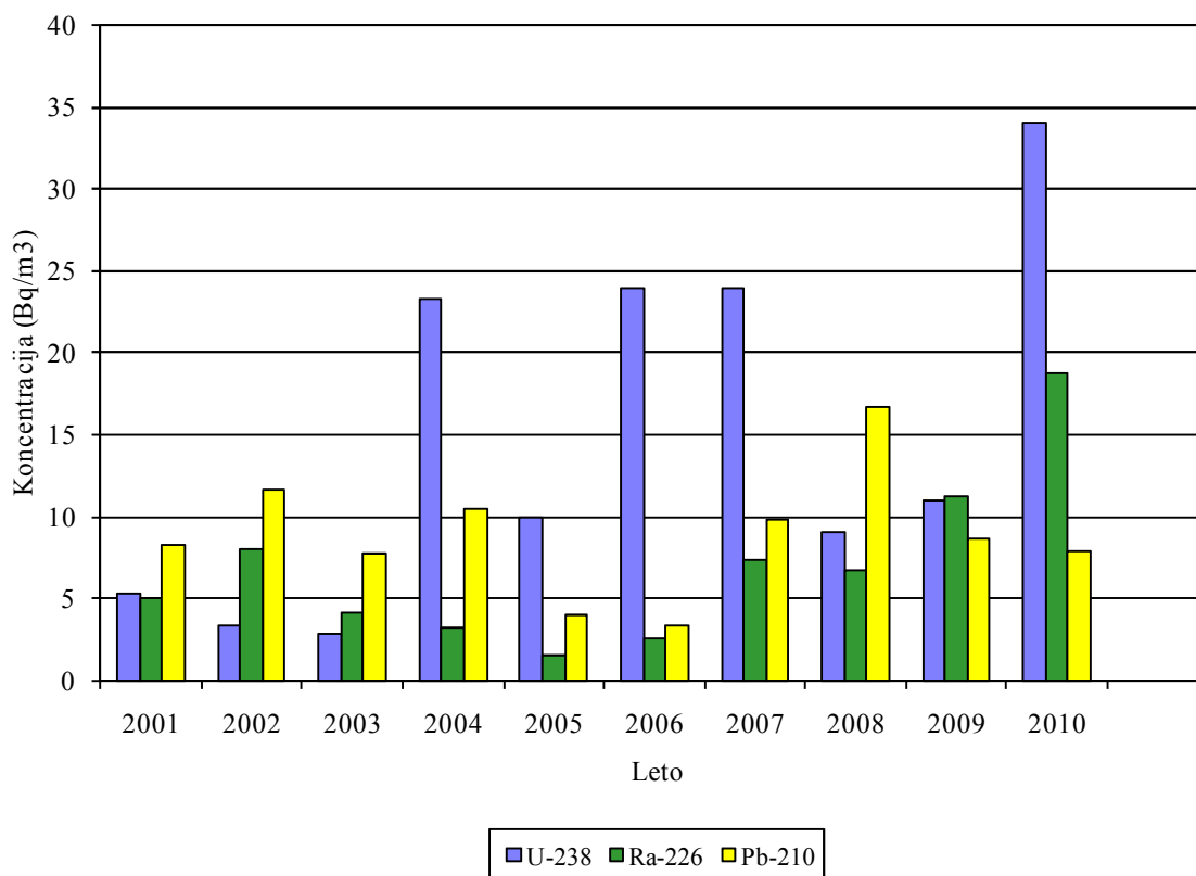
Slika 18: Koncentracije U-238, Ra-226 in Pb-210 v vodnjaku na domačiji Drmota
