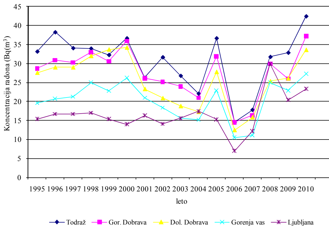
Slika 8: Povprečne letne koncentracije radona v okolici RŽV, merjeno z ogljenimi adsorberji
