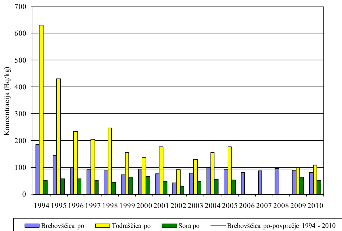
Slika 20: Koncentracija Ra-226 v sedimentih voda v okolici RŽV
