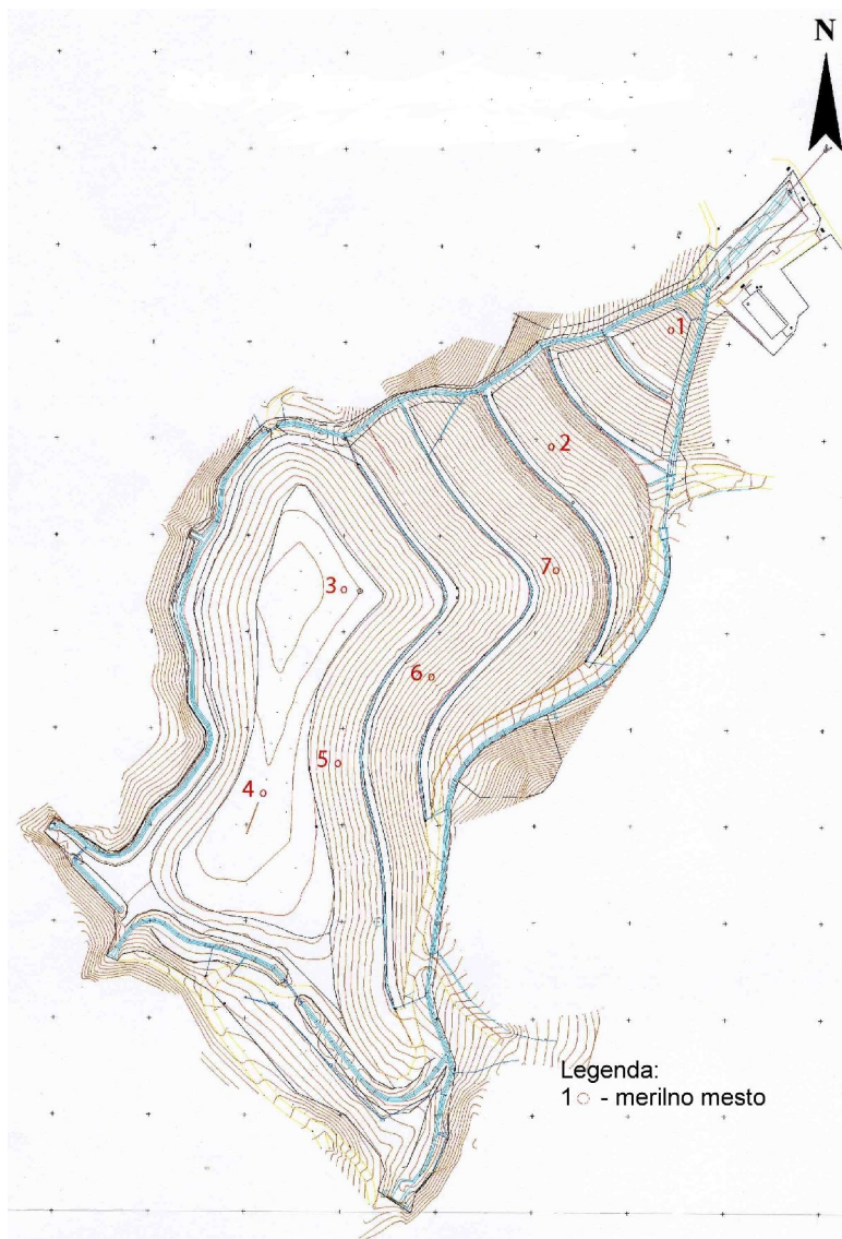
Slika 9: Lokacije meritev ekshalacije radona na odlagališču Jazbec. Najvišje vrednosti so izmerjene na lokaciji št. 1, najnižje na lokaciji št. 3.
