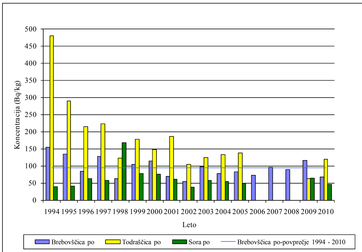
Slika 21: Koncentracija Pb-210 v sedimentih voda v okolici RŽV
