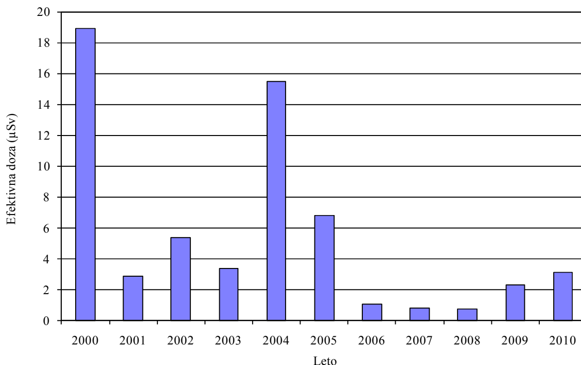
Slika 23: Letne efektivne doze v okolici RŽV zaradi vdihavanja dolgoživih radionuklidov v zraku za odraslega prebivalca
