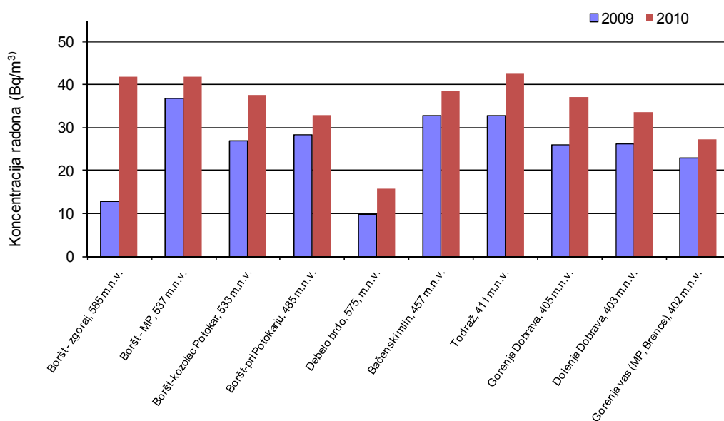
Slika 12: Višinski profil koncentracije radona po dolini Todraščice, merjeno z ogljenimi adsorberji
