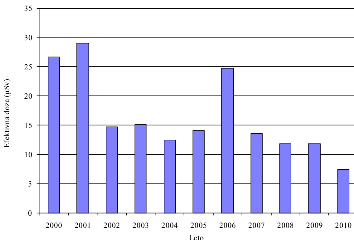
Slika 25: Letne efektivne doze zaradi pitja vode (Brebovščica) za odraslega prebivalca iz okolice RŽV
