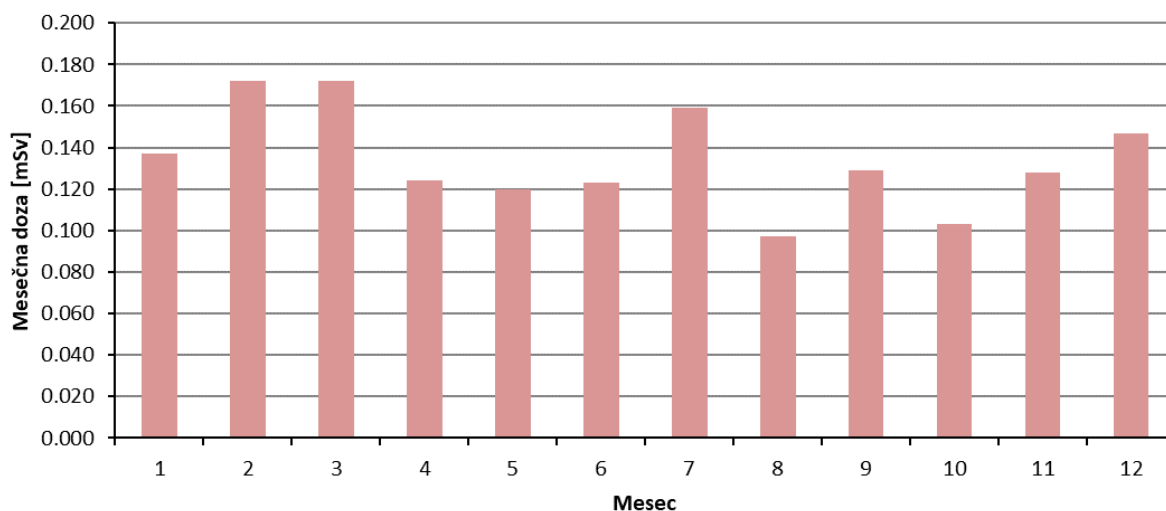
Slika 3: Mesečne doze TLD na izpuhu iz reaktorja v letu 2018 (Oznaka: 1.7D)
