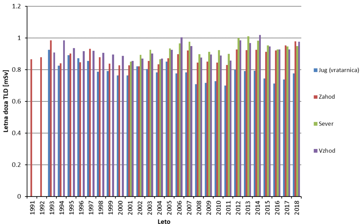
Slika 5: Letne doze TLD na merilnih točkah v obdobju 1991 – 2018
