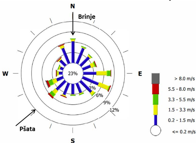
Slika 11: Roža vetrov za leto 2018, osrednji del predstavlja brezvetrje (23 %)
