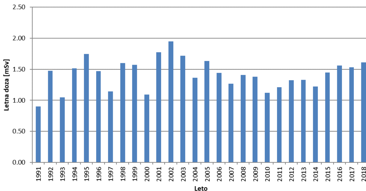
Slika 2: Letne doze TLD na izpuhu iz reaktorja za obdobje 1991 – 2018
