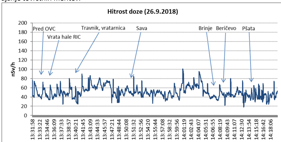
Slika 8: Meritve hitrosti doze na krožni poti v okolici Reaktorskega centra (26.9.2018) s scintilacijsko sondo Automess 6150AD-b/H)
