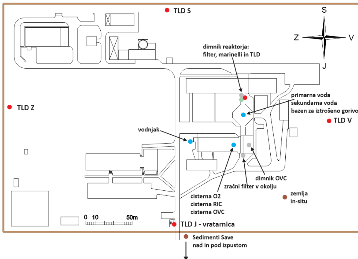
Slika 1: Vzorčevalne lokacije na Reaktorskem centru v letu 2018
