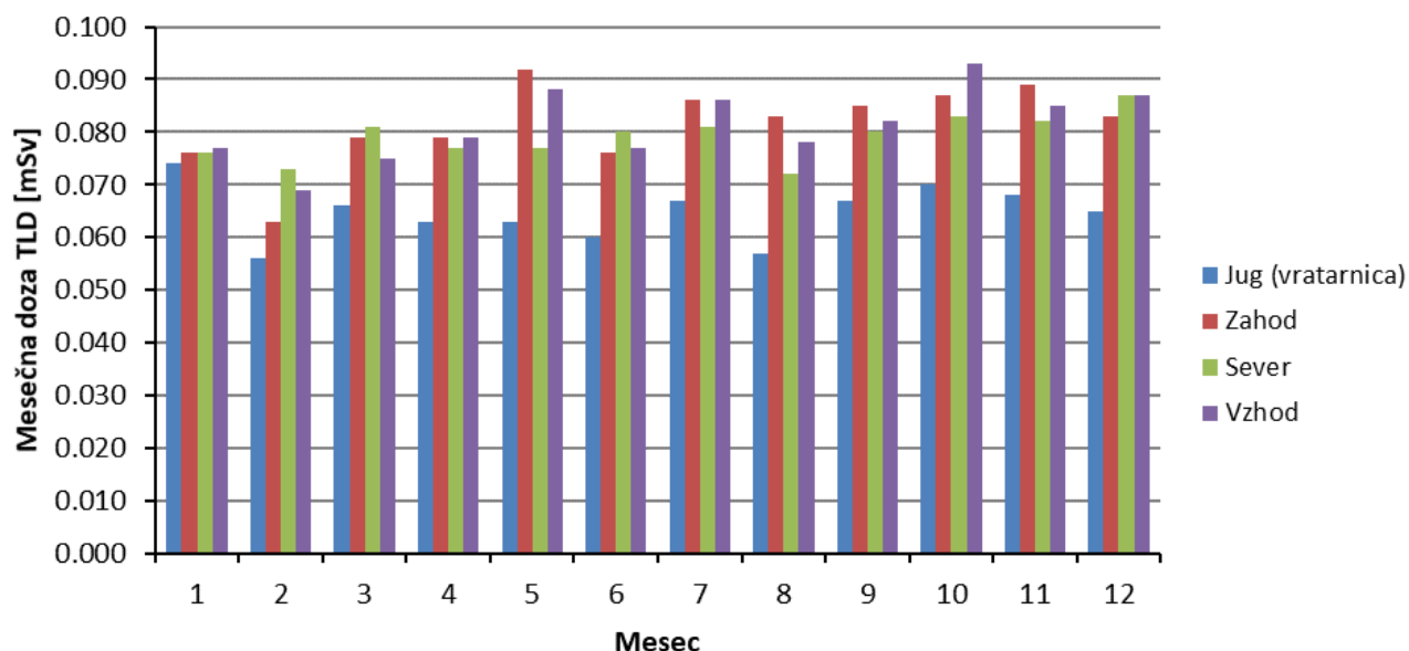
Slika 4: Mesečne doze TLD na merilnih točkah v letu 2018 (Oznaka 2.6D – 2.9D)
