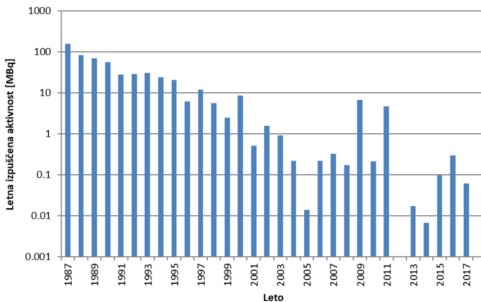
Slika 12: Letne izpuščene aktivnosti iz cisterne odseka O-2 v obdobju 1987-2018
