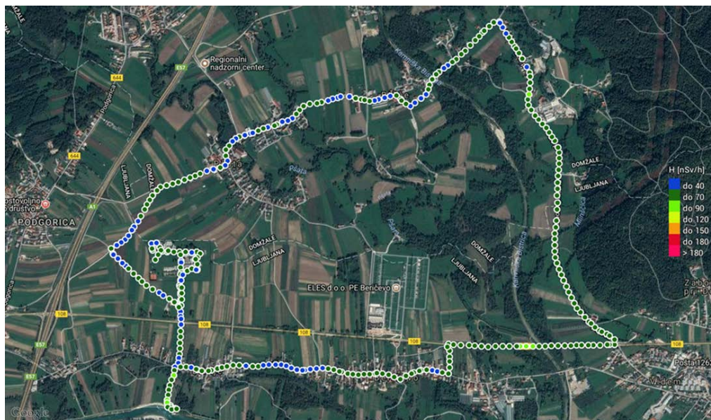
Slika 9: Lokacija meritev hitrosti doze na krožni poti v okolici Reaktorskega centra (26. 9. 2018)
