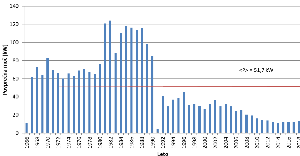
Slika 10: Povprečna obratovalna moč reaktorja TRIGA v obdobju 1966-2018, <P> je povprečje za celotno življenjsko obdobje reaktorja TRIGE
