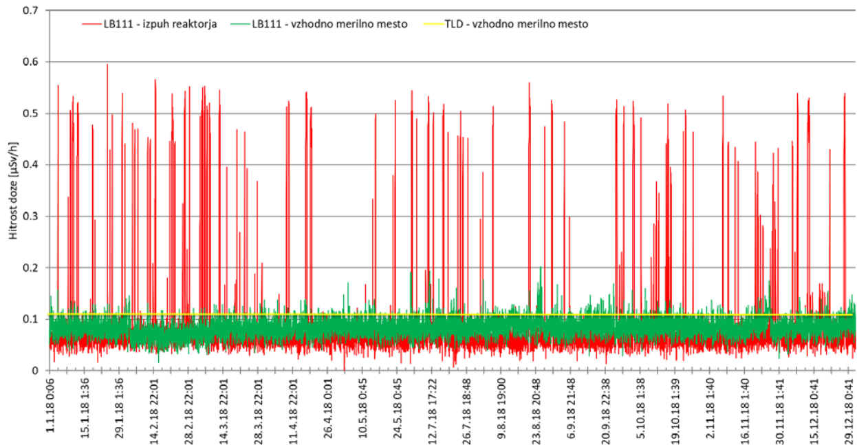
Slika 6: Hitrost doze na vzhodni merilni točki in na izpuhu v letu 2018 (kontinuirni merilnik Berthold LB111 in TLD) (Oznaka: 1.6HD)
